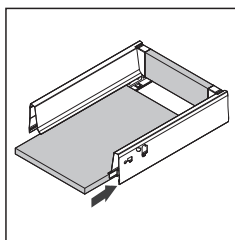
Parte inferior Bottom assembly
