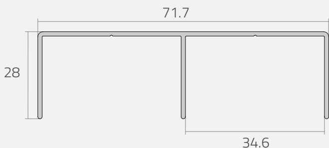
Vista de corte perfil superior
