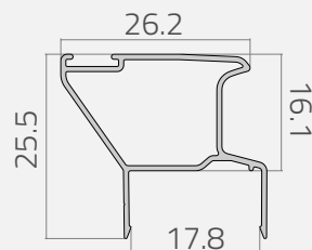
Vista de corte de la manija
