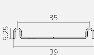
Vista de corte perfil inferior
