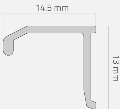
Vista de corte del perfil
