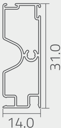
Vista de sección del perfil
